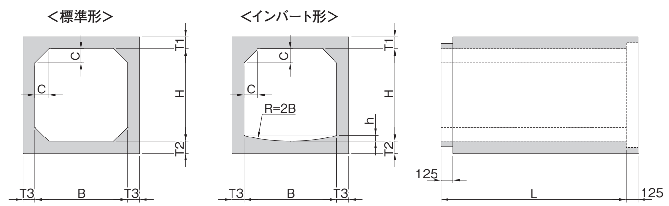
●RCボックスカルバート (単位: mm)
